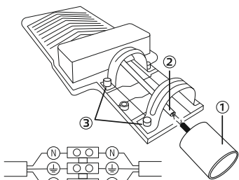
Рис. 1. Монтаж светильника
